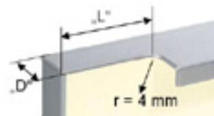
Vermassung der Fräsung «elegance»
