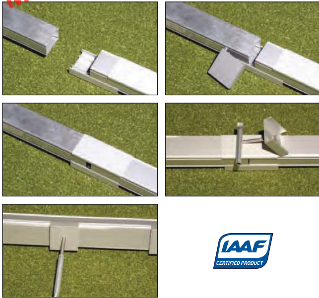
Laufbahnbegrenzung (Zarge), komplett aus Aluminium gefertigt, mit IAAF-Zertifikat
