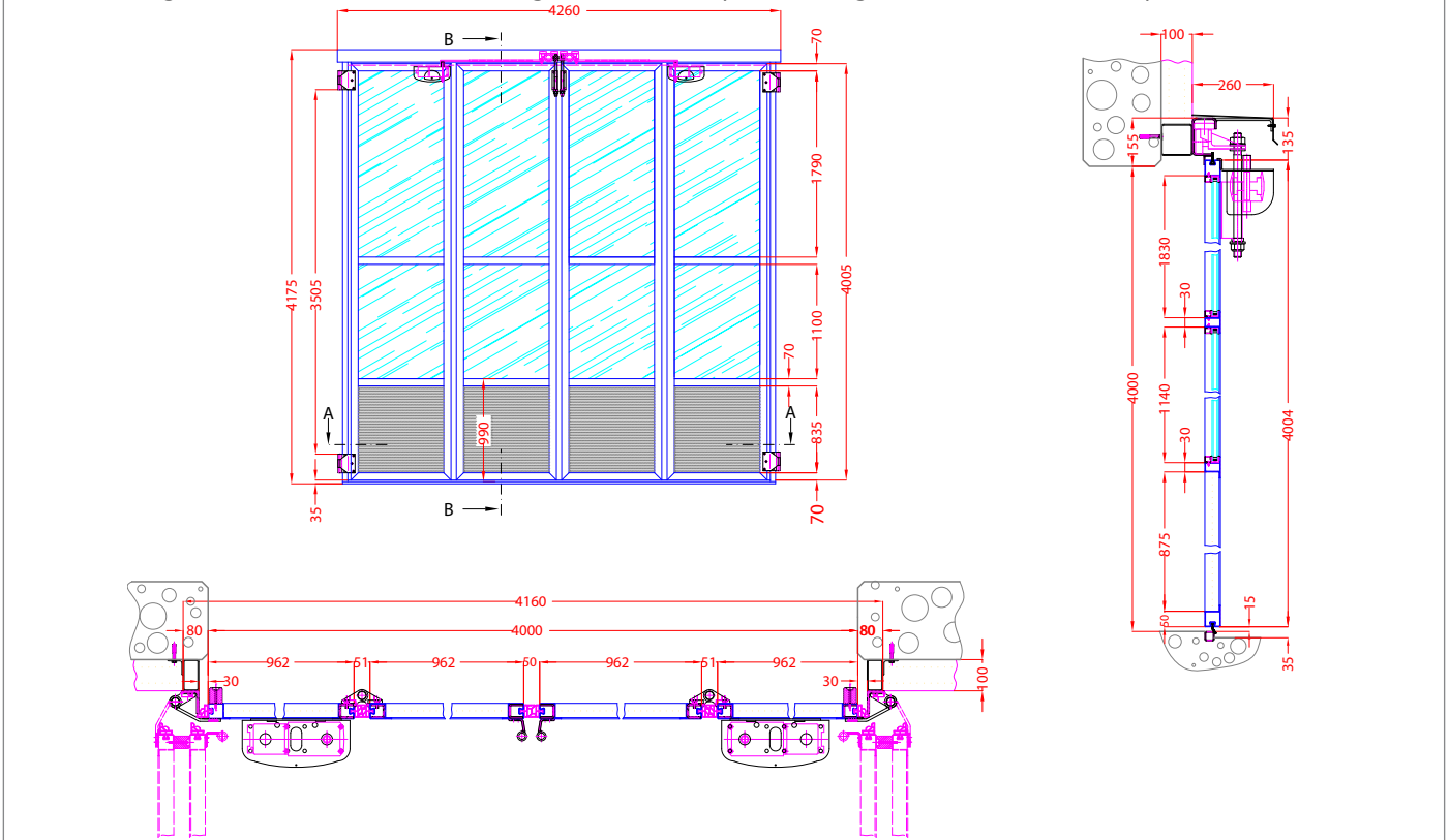
FT - Austragend mit Automat 2+2 Flügel - FT with special hinges with automatic operator 2+2 sections
