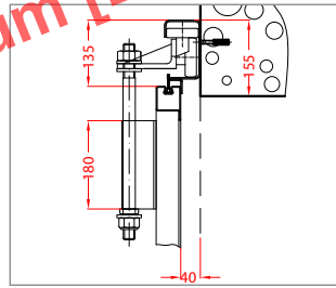
Laufschienenprofil auf Laibung
