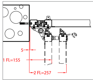
Stockteil in Laibung
