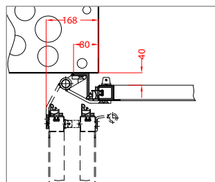
Stockteil austragend
