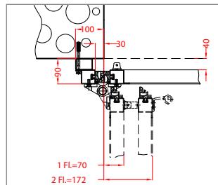
Stockteil 90° / 180°
