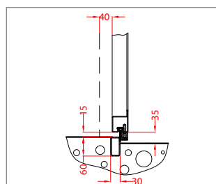
Anschlag Bodenschiene
