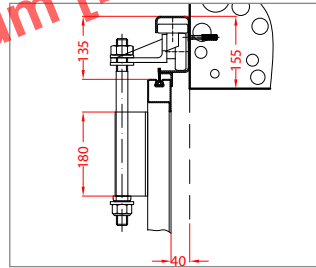
Laufschiene auf Laibung running rail profile – on embrasure
