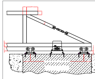
Rollenböcke mit Automat
