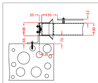
Einlaufhalterung
